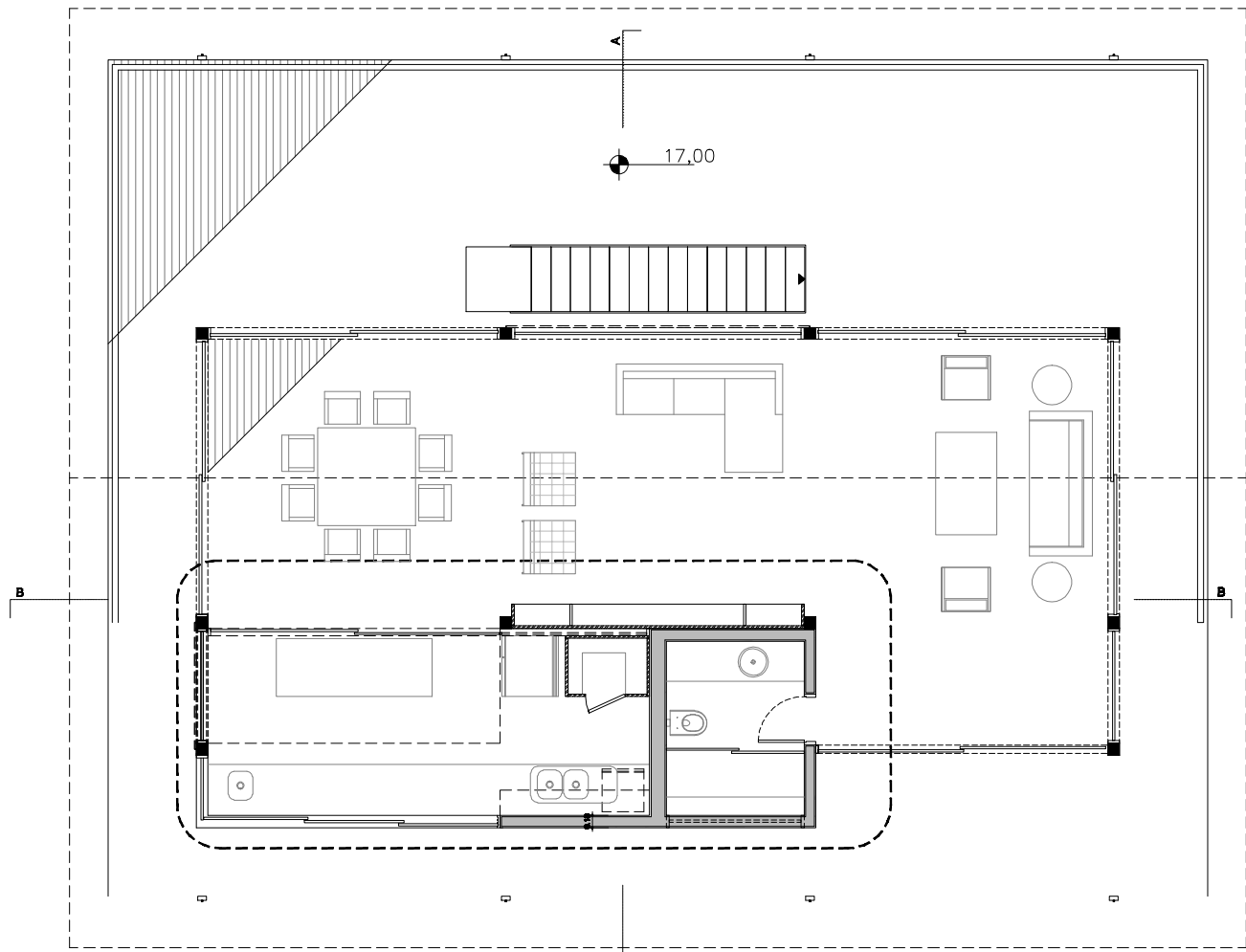
PLANTA PAVIMENTO SUPERIOR ESC. 1:100
