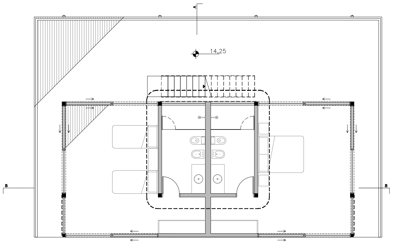
PLANTA PAVIMENTO SUPERIOR ESC. 1:100
